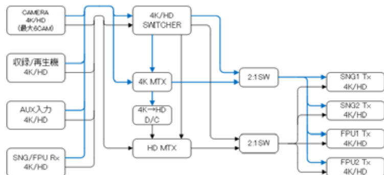
映像システム概念図
